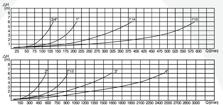
DIAGRAMMA PERDITE DI CARICO (3/4"÷4")
