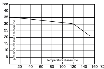
DIAGRAMMA DI PRESSIONE - TEMPERATURA (1/4"÷1/2")
