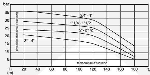
DIAGRAMMA DI PRESSIONE - TEMPERATURA (3/4"÷4")
