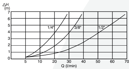
DIAGRAMMA PERDITE DI CARICO (1/4"÷1/2")
